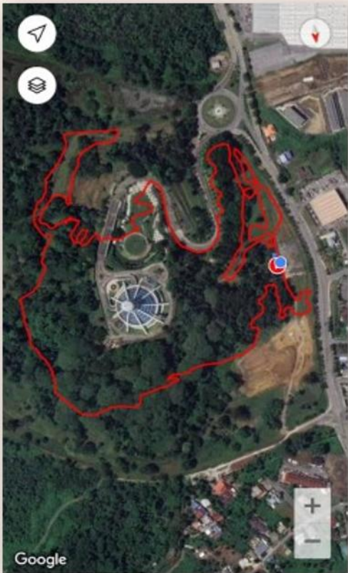
XCO 3.67 KM
